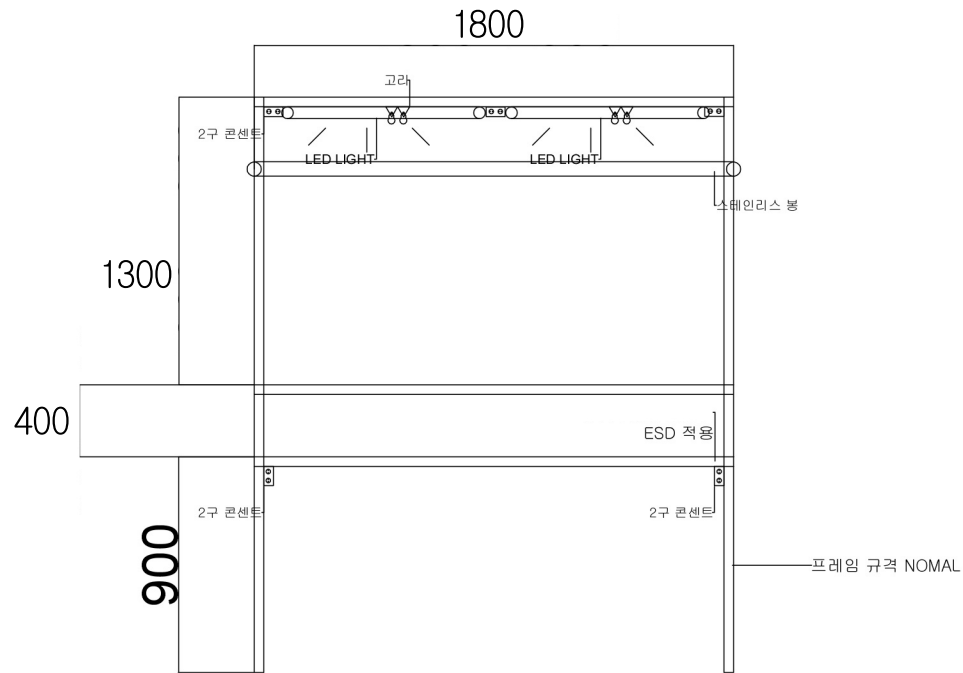
정면도
