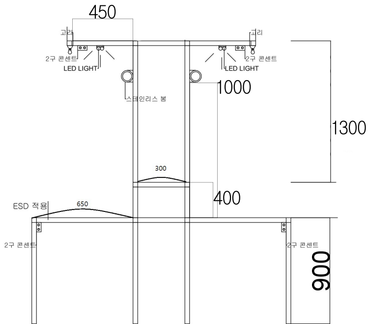
단면도
